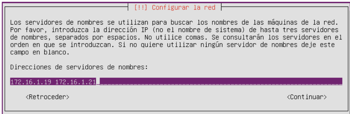
Ilustración 9 Pantalla de Inserción de las IP de los Servidores de DNS
